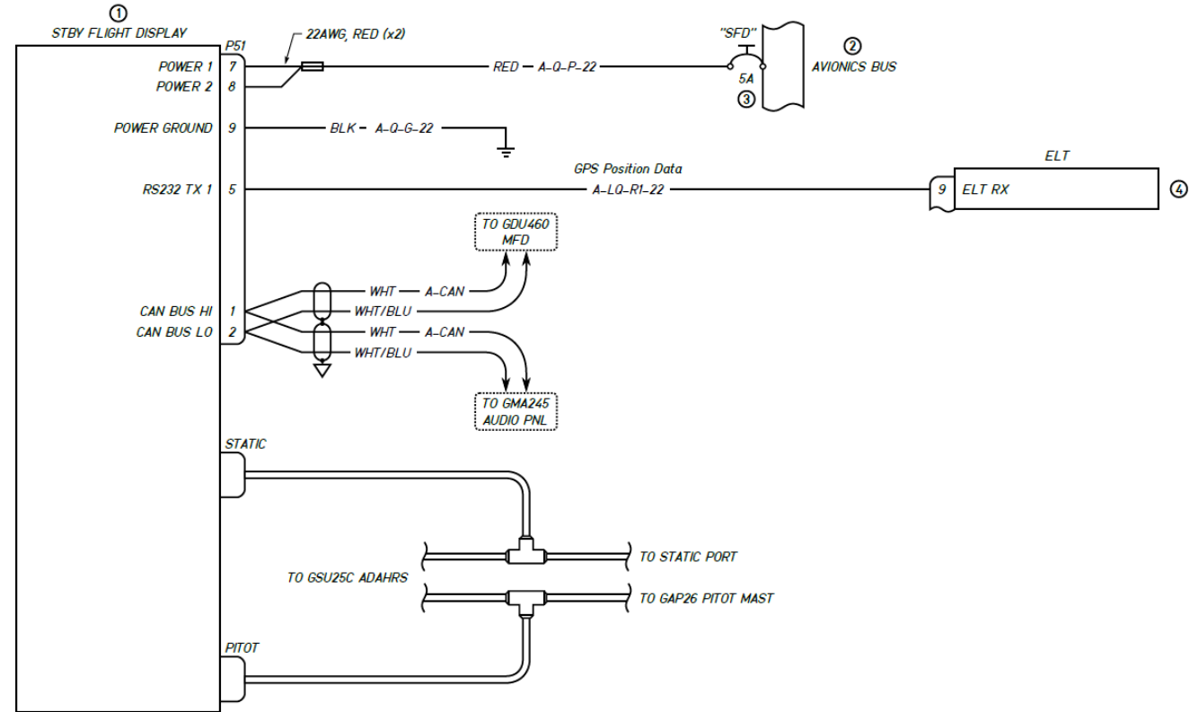
Figura 9.2.13.1. Diagrama G5
