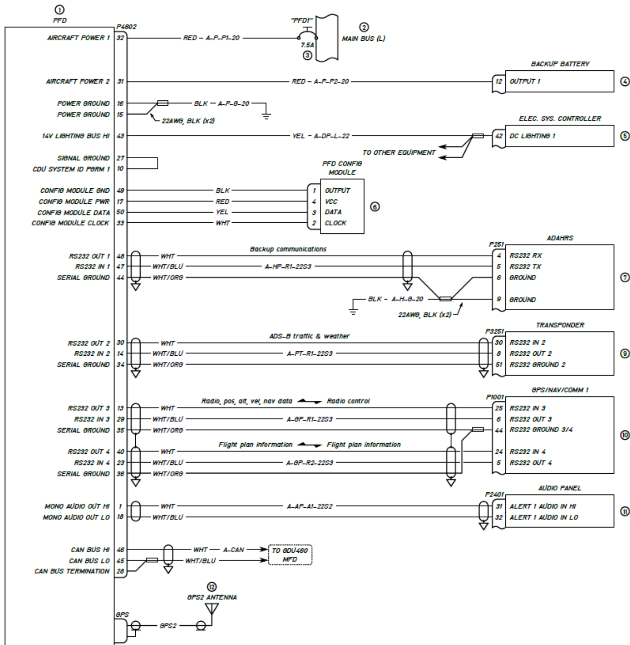
Figura 9.2.3.1. Diagrama GDU 460 PFD
