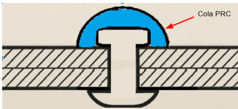
Figura 2.4.25.2. Reparo de rebite único.
