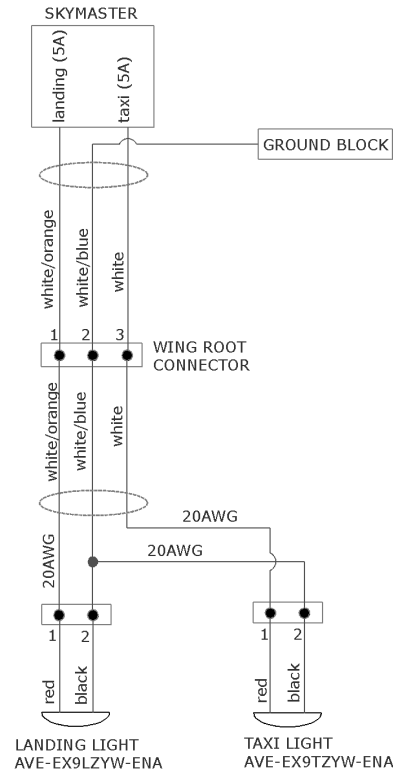
Figura 9.10.1. Diagrama das Luzes de Pouso / Taxi.
