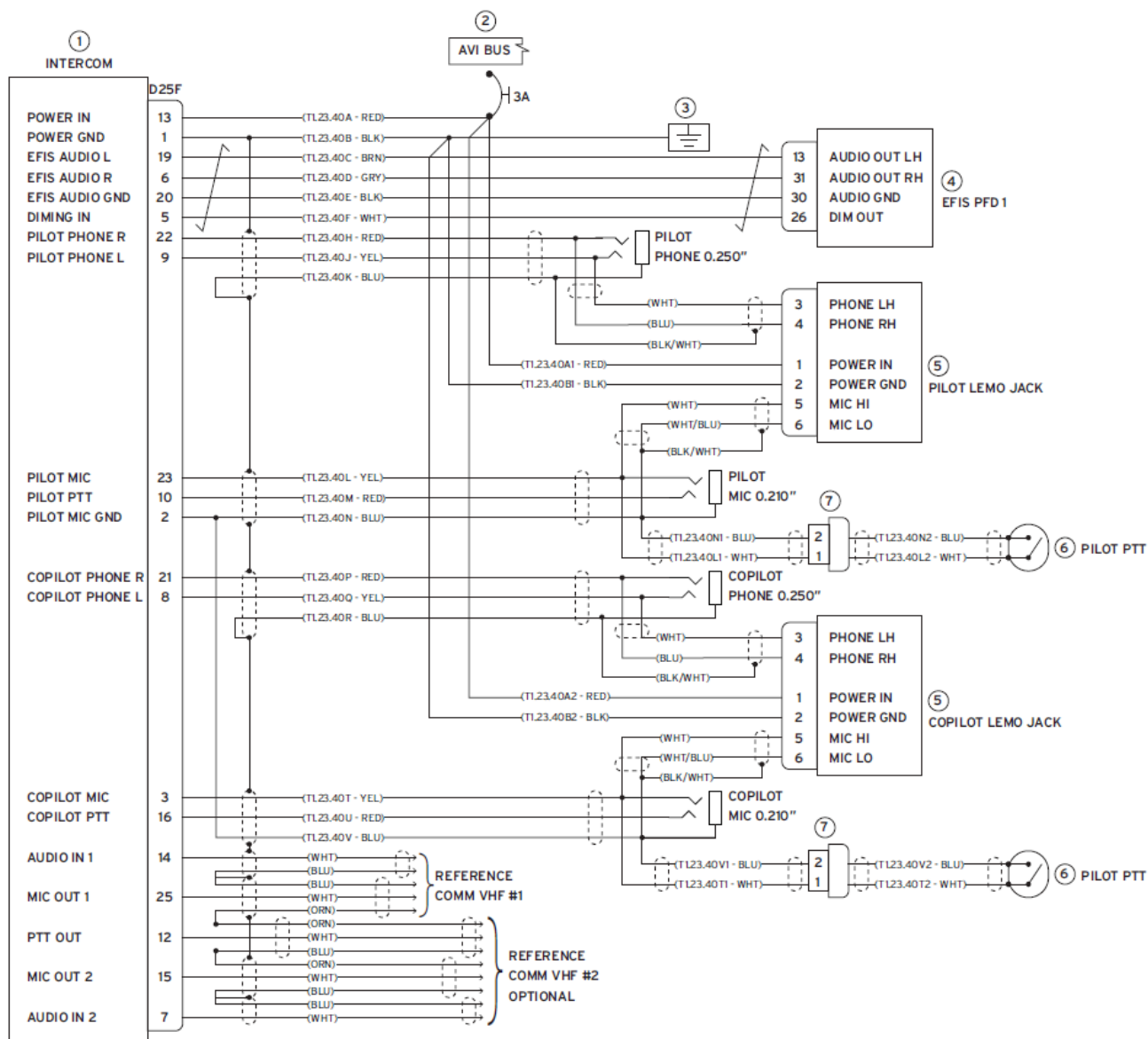
Figura 9.9.1. Diagrama do Intercom.
