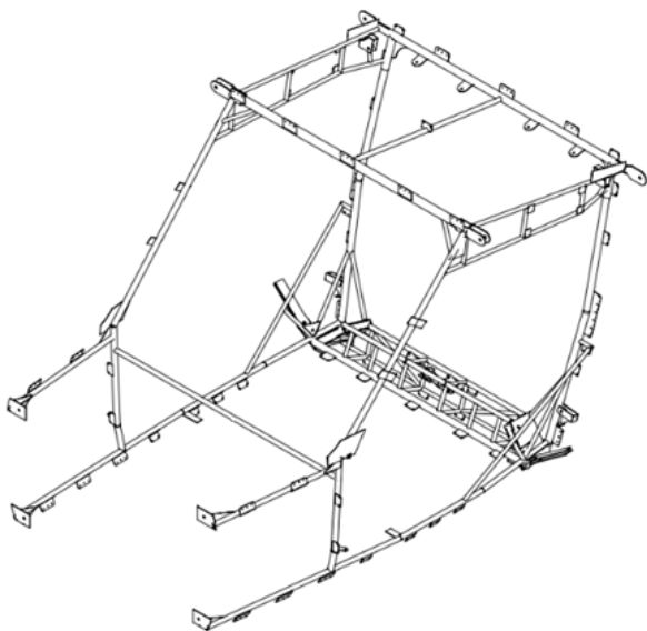
Figura 3.6.2.1. Estrutura de Treliça do Cockpit.
