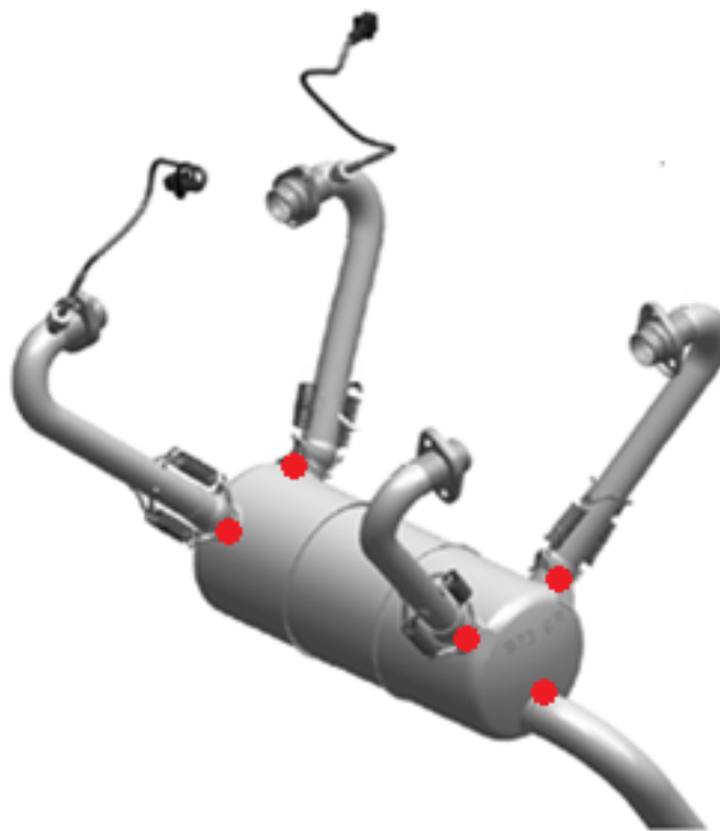
Figura 2.4.17.1. Pontos de Inspeção de Exaustão.
