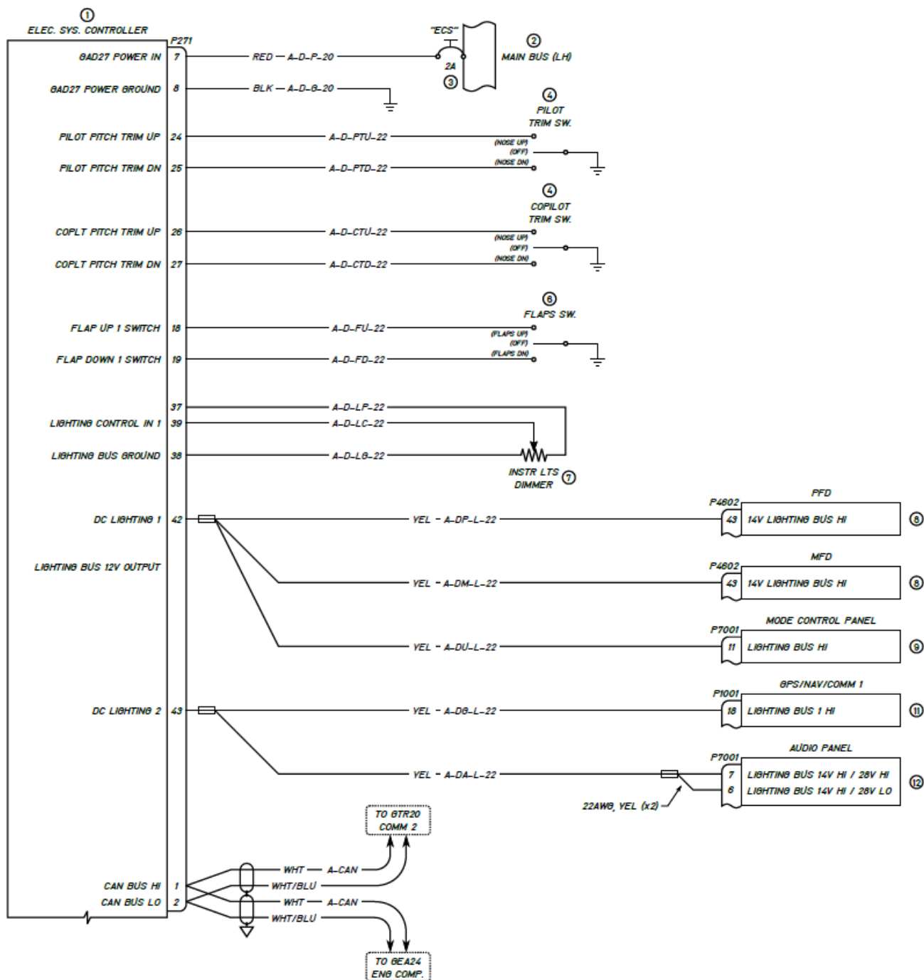
Figura 9.2.8.1. Diagrama GAD 27
