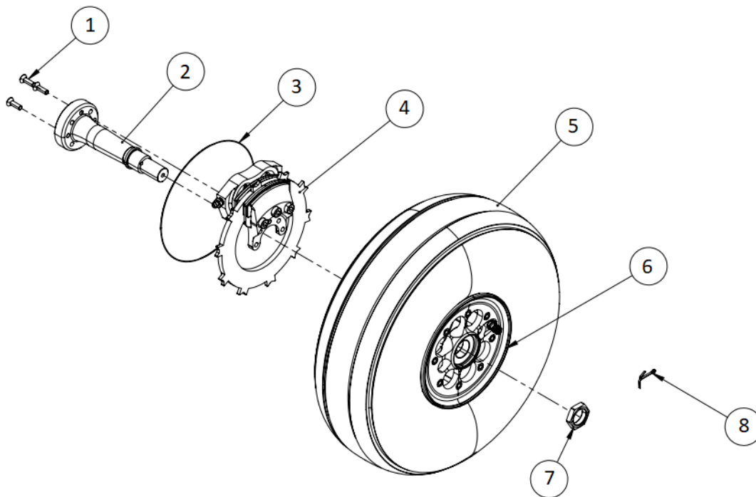
Figura 3.5.1.1 Conjunto do trem de pouso principal.
