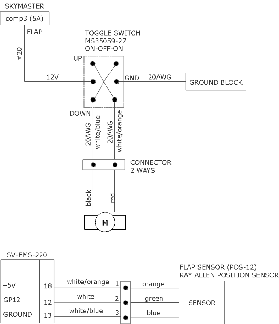
Figura 9.8.1. Diagrama do Flap.
