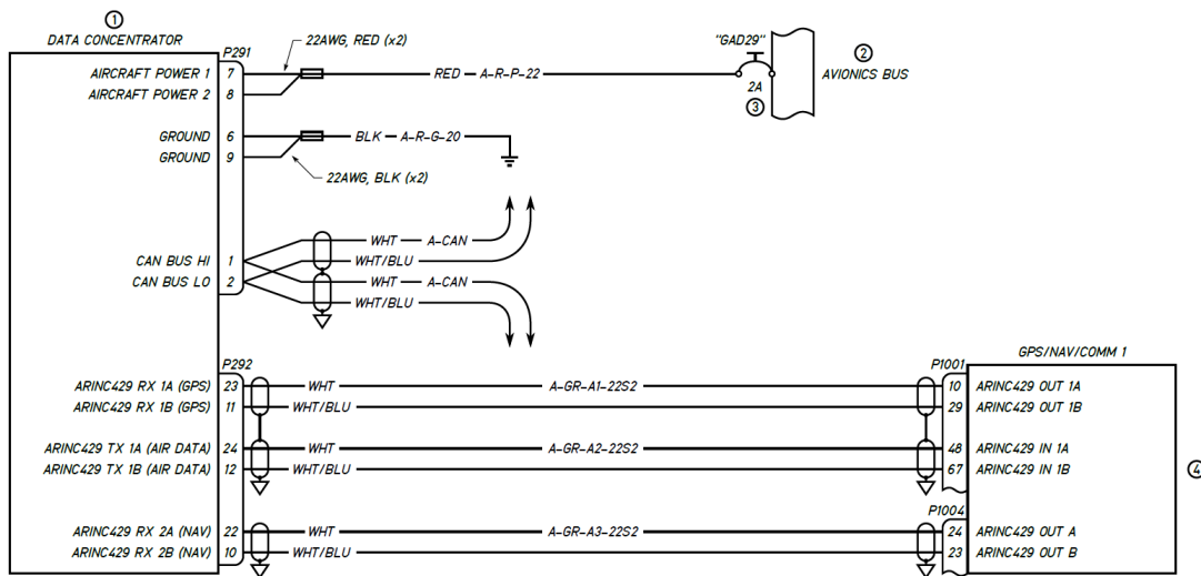
Figura 9.2.14.1. Diagrama GAD 29
