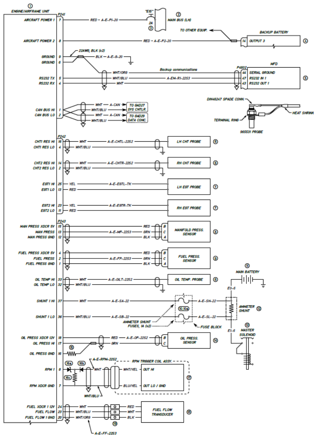
Figura 9.2.7.1. Diagrama GEA 24
