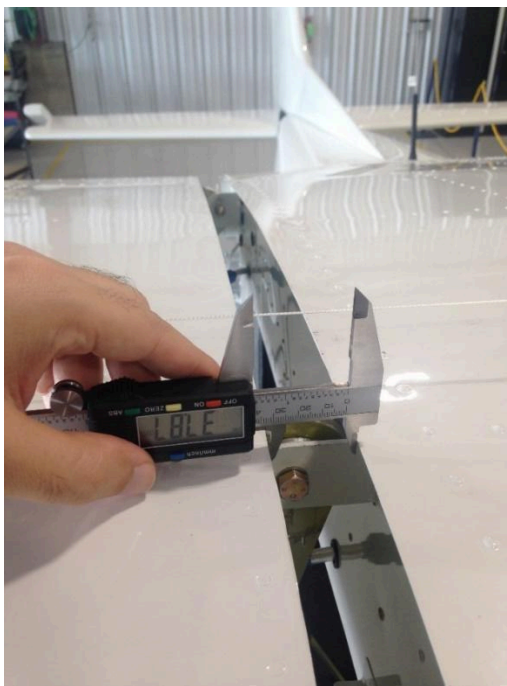
Figura 2.1.5. Espaço entre a fuselagem e as asas.
