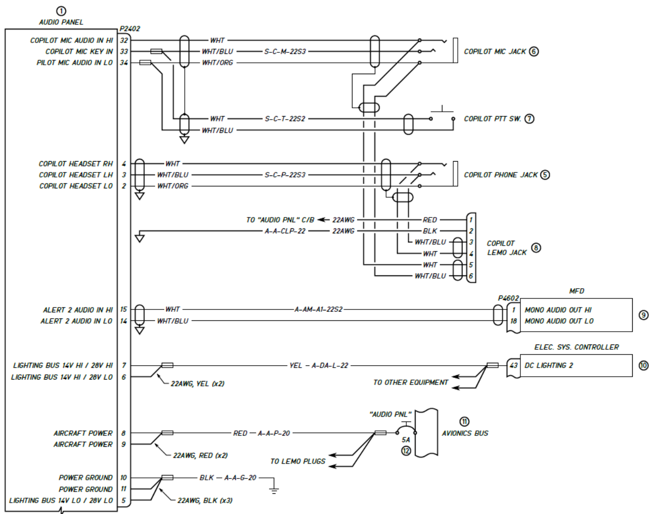
Figura 9.2.10.1. Diagrama GMA 245 PAINEL DE ÁUDIO (continuação)
