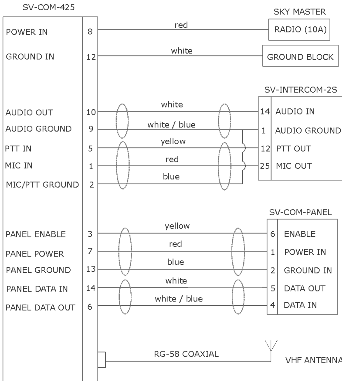
Figura 9.5.1. Diagrama do Rádio 1.
