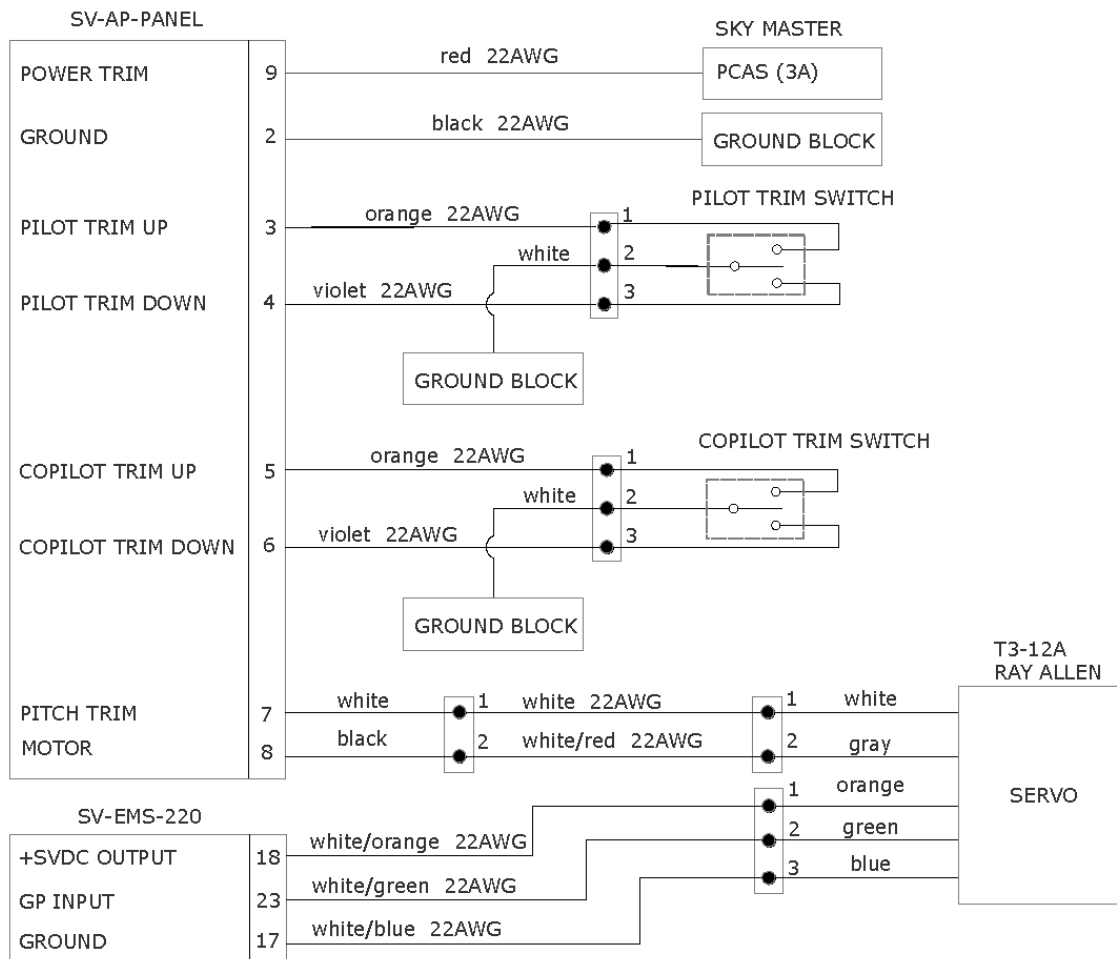
Figura 9.2.1. Auto Trim.
